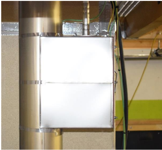
Montierter Nachrüstsatz
