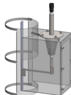
OekoTube-Inside Rauchrohrmontage
