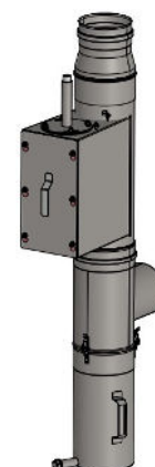
Anschlussset T-Stück, Staubbehälter L310mm, Reduktion und 2 Klemmbänder
