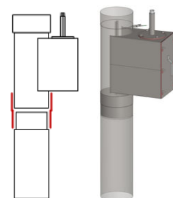
Übergang auf eingezogenes Rauchrohr, enge Steckseite
